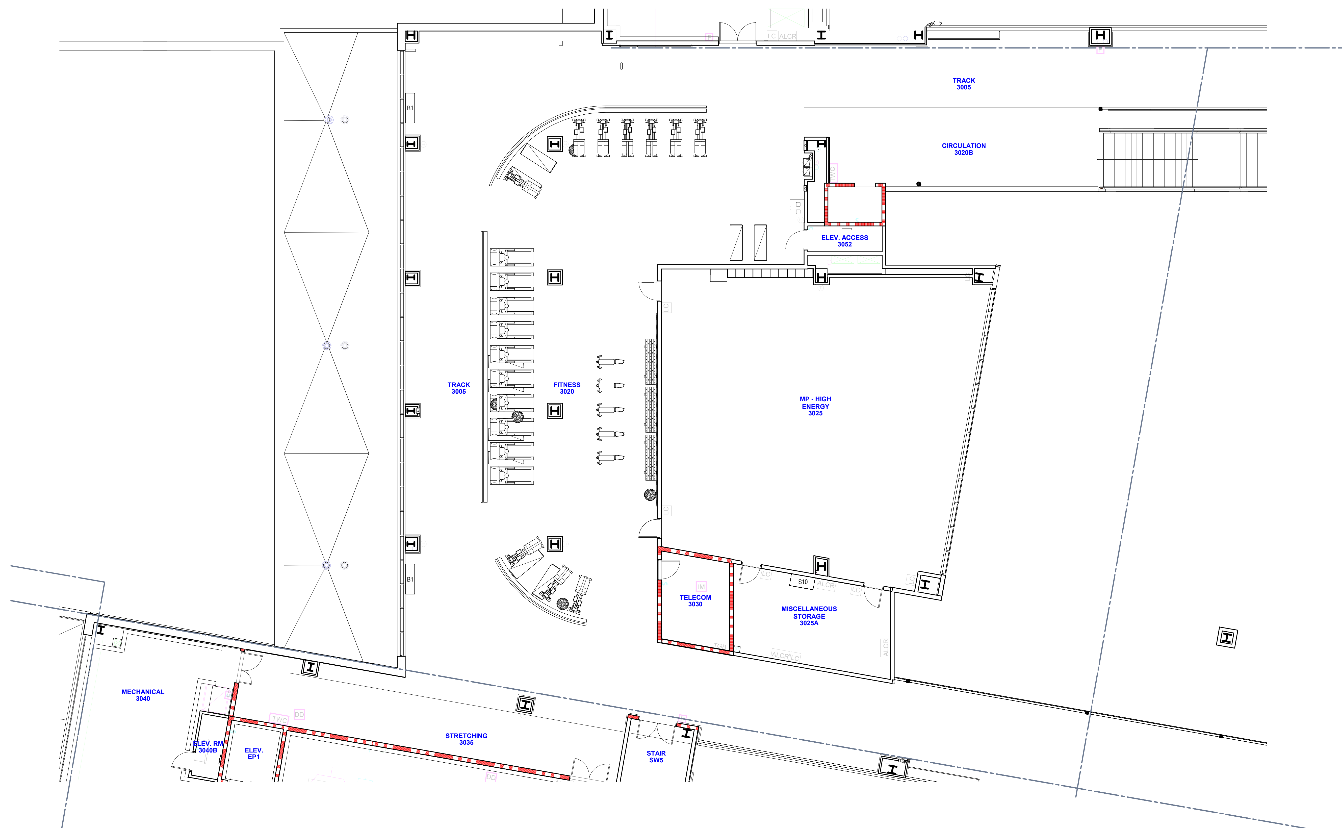
1 FURNITURE PLAN - MEZZANINE LEVEL - AREA 3 A-1016 SCALE: 1/8" = 1'-0"
