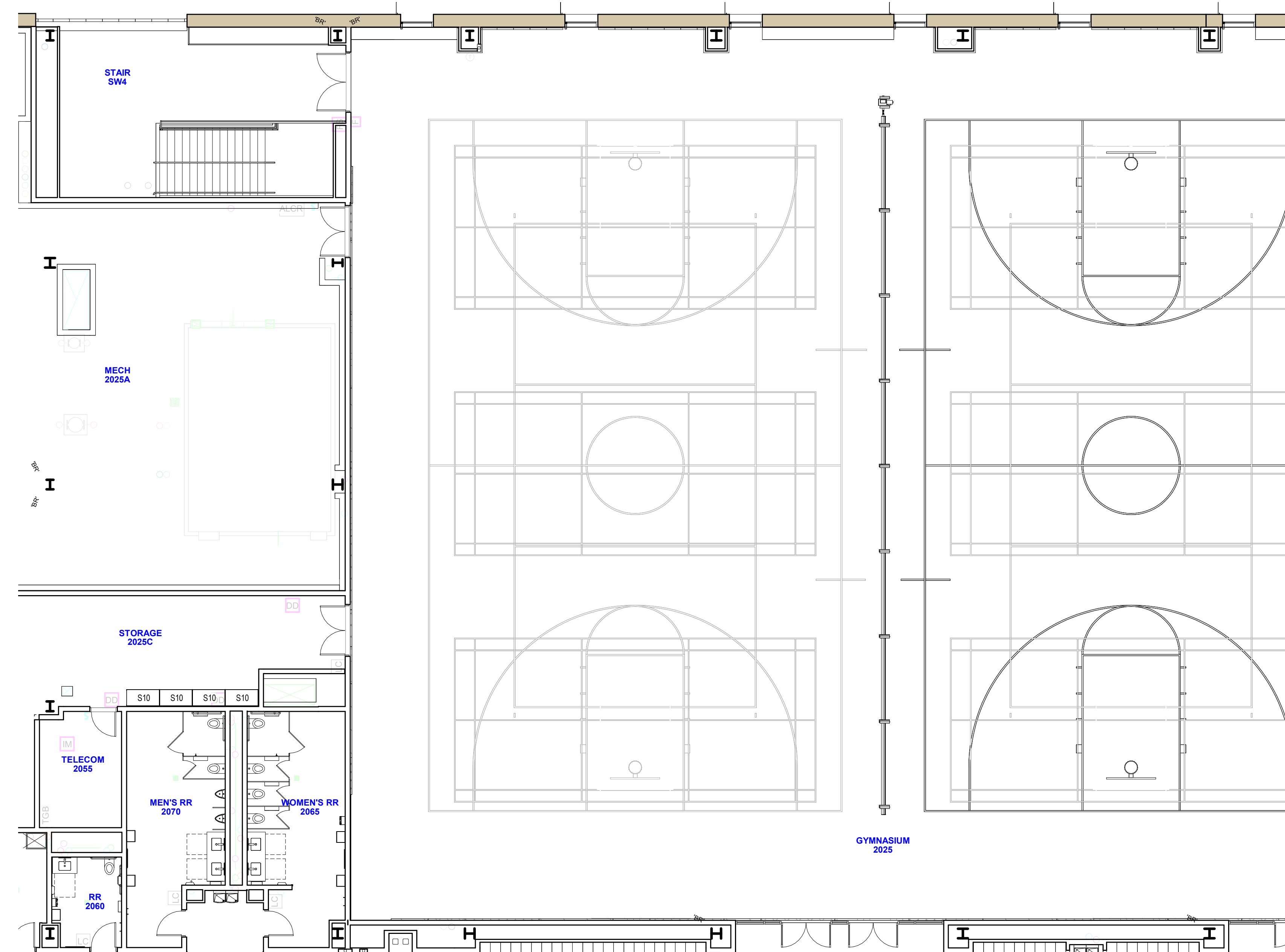
1 FURNITURE PLAN - LEVEL 02 - AREA 5 A-1015 SCALE: 1/8" = 1'-0"
